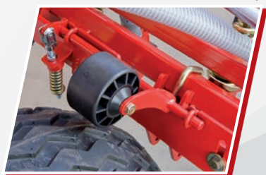
Stop automatico della distribuzione in fase di manovra a fine campo
